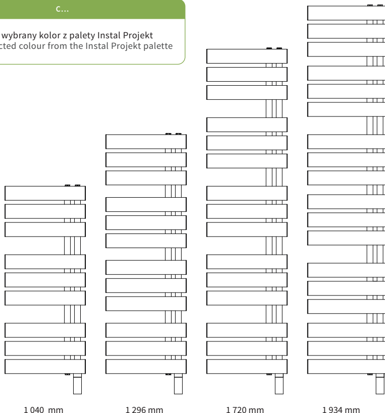
UKŁAD GRZEJNIKA PRZY WYSOKOŚCI: radiator shape and design with the height:
